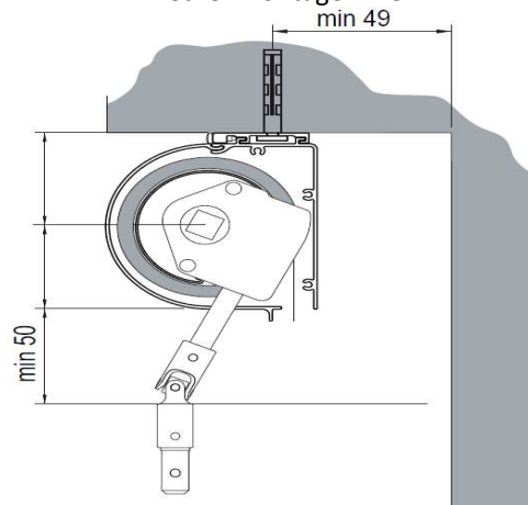
Deckenmontage Innen
