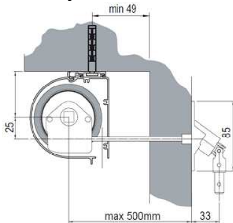
Deckenmontage Außen mit Wanddurchführung
