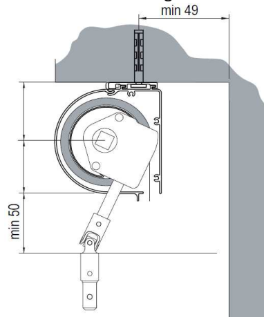
Deckenmontage Innen
