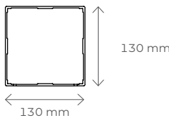
Pfosten – Querschnitt
