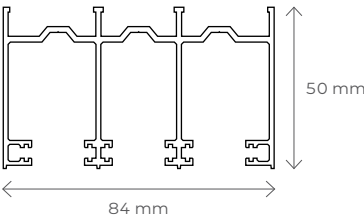
Oberprofil – Querschnitt
