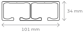
Untere zweiläufige Führungsschiene – Querschnitt
