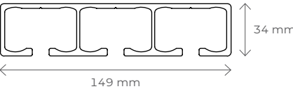
Untere dreiläufige Führungsschiene – Querschnitt
