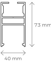
Oberer Rahmen – Querschnitt
