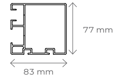
Führungsschiene – Querschnitt
