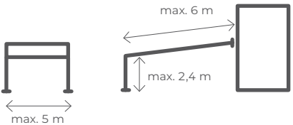
Pergolaabmessungen
