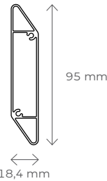
Obere dreiläufige Führungsschiene – Querschnitt
