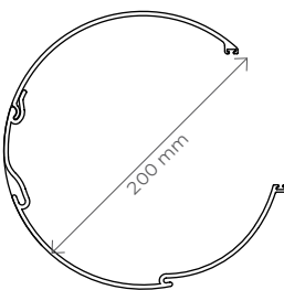
Kassette – Querschnitt
