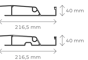
Pfosten – Querschnitt
