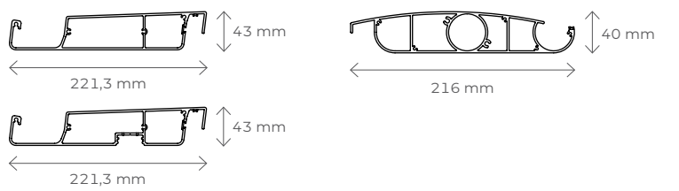
Träger mit integriertem Motor – Querschnitt Träger mit sichtbarem Motor – Querschnitt
