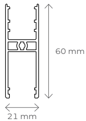
Unterer Rahmen – Querschnitt
