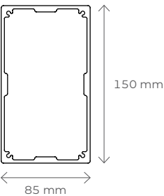
Pfosten – Querschnitt
