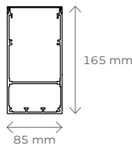
Träger – Querschnitt
