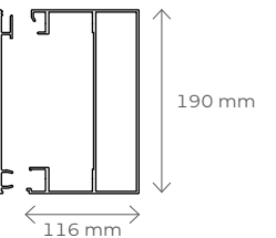
Träger – Querschnitt
