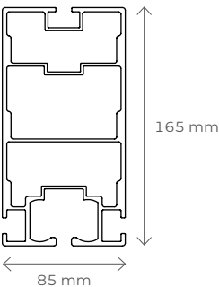
Führungsschiene – Querschnitt
