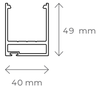
Seitlicher und unterer Rahmen – Querschnitt
