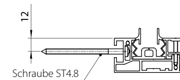
Montage auf den Rahmen
